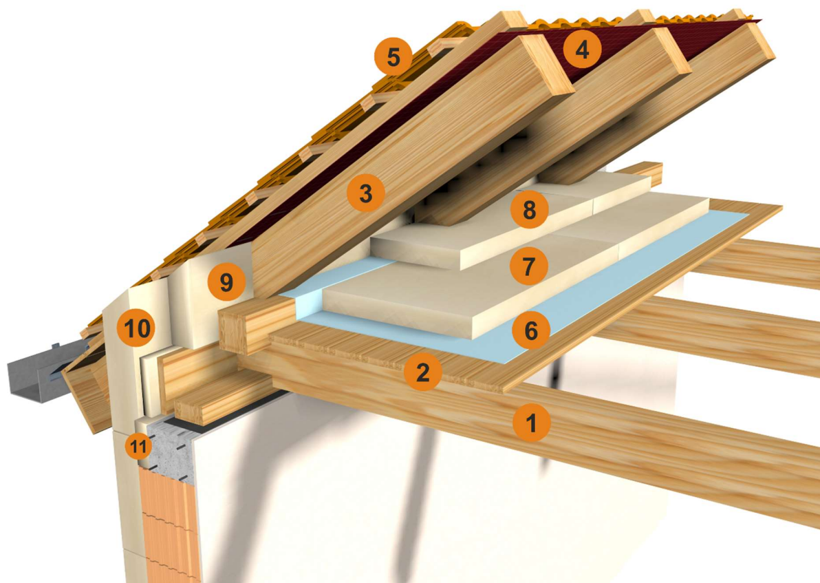
Padlástéri födém hőszigetelése – fa teherhordó szerkezettel, alulról látszó gerendázattal – MF/Therm PIR
