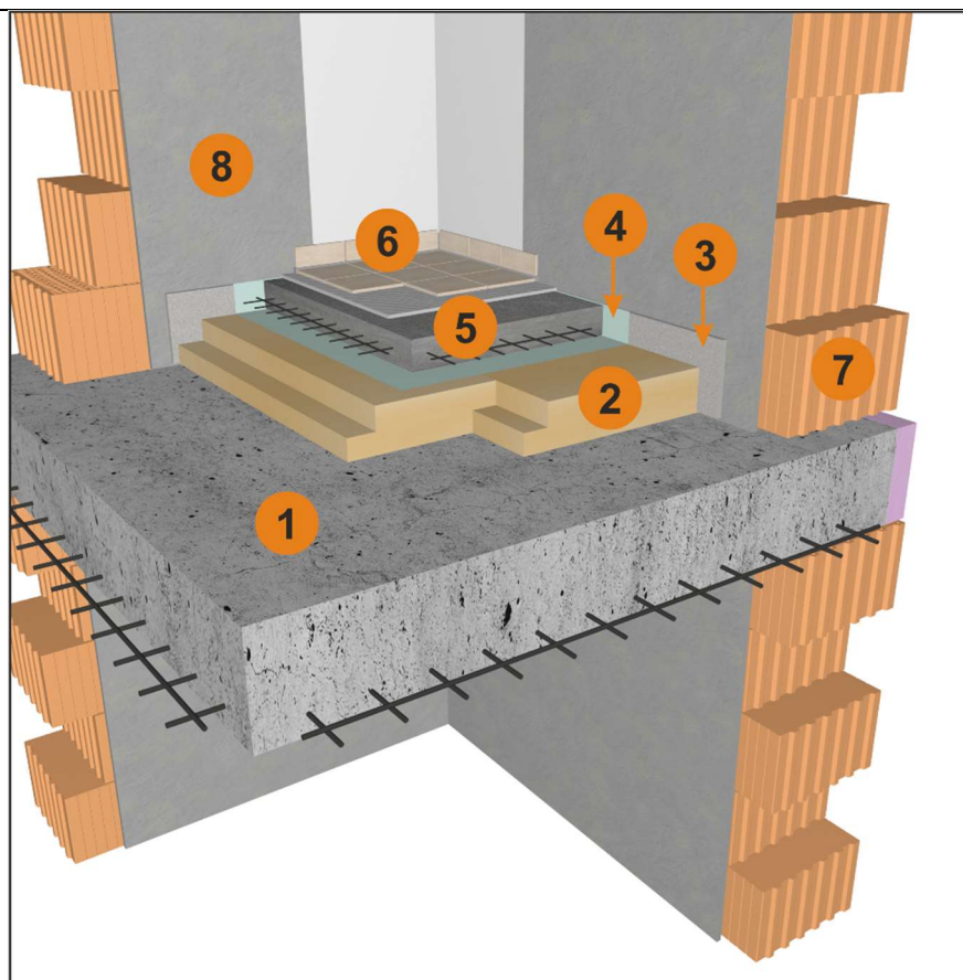
Közbenső fűtetlen padló hőszigetelése – vasbeton teherhordó szerkezettel
