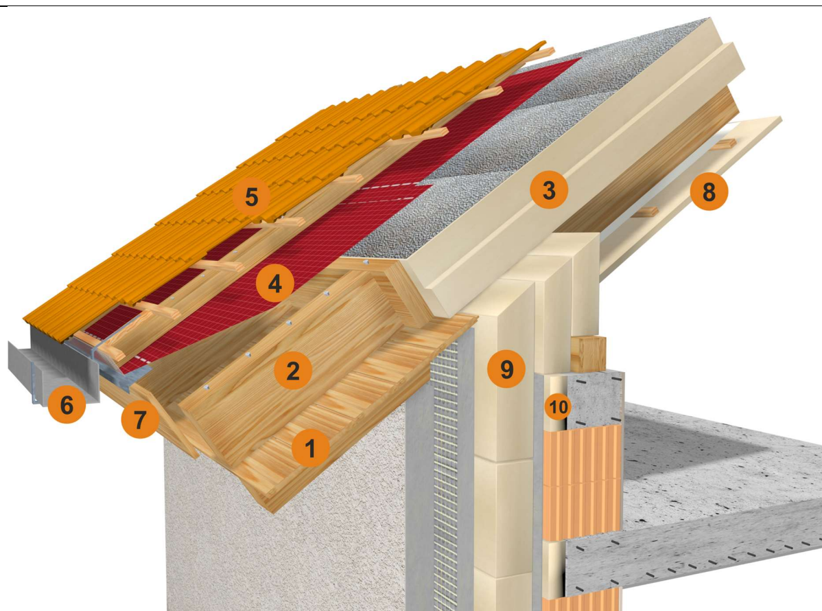
Magastető, külső oldali és közbelső hőszigeteléssel, tetőtér beépítésnél, deszka aljzat nélkül (ERESZ RÉSZLET)
