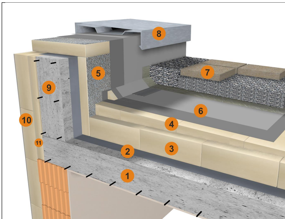
Egyenes rétegrendű terasztető, vasbeton aljaton, hőszigetelő lejtésképzéssel - bitumenes lemezes vízszigeteléssel (ATTIKA RÉSZLET)
