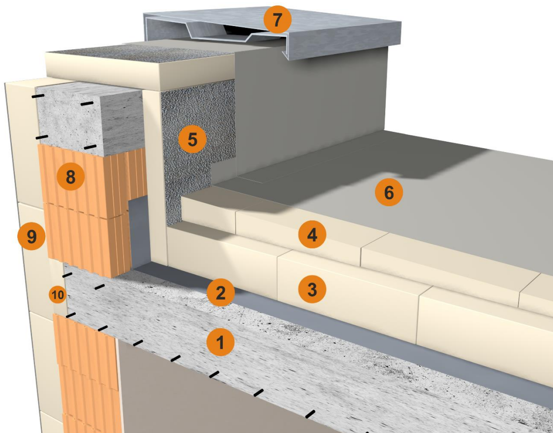
Egyenes rétegrendű nem járható lapostető, vasbeton aljzaton, hőszigetelő lejtésképzéssel - műanyag lemezes vízszigeteléssel (ATTIKA RÉSZLET)
